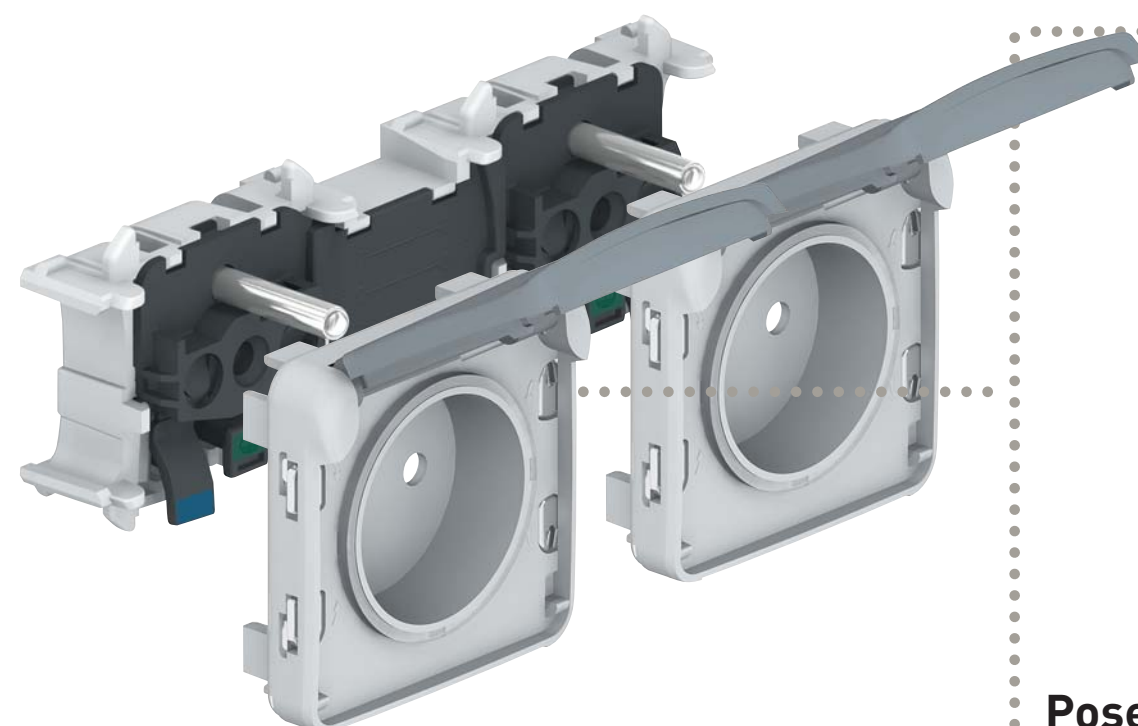
Mécanisme prise double précâblée* (horizontale ou verticale). Existe aussi en triple horizontale.
